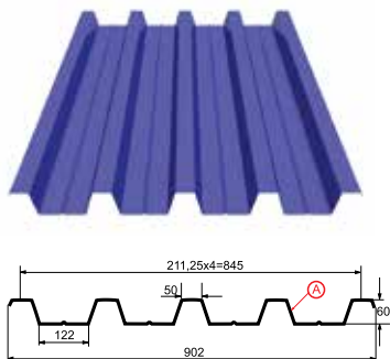
Профилированный лист Н-60x845-А Толщина материала 0.5 - 1.0 мм
