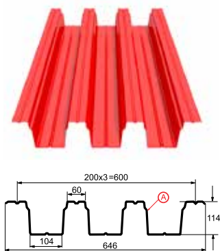
Профилированный лист Н-114x600-А Толщина материала 0.7 - 1.0 мм
