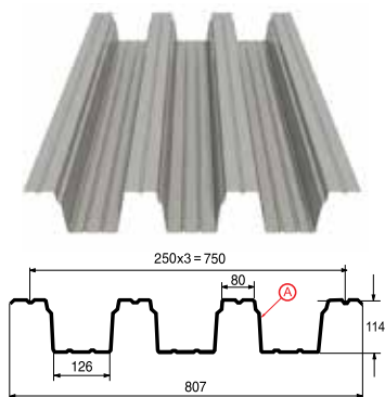
Профилированный лист Н-114x750-А Толщина материала 0.7 - 1.0 мм
