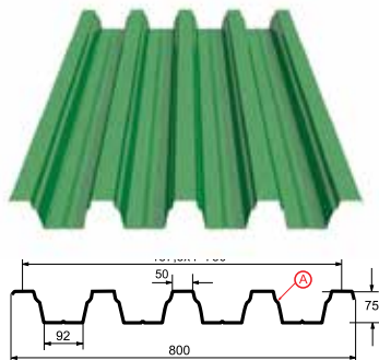
Профилированный лист Н-75x750-А Толщина материала 0.65 - 1.0 мм
